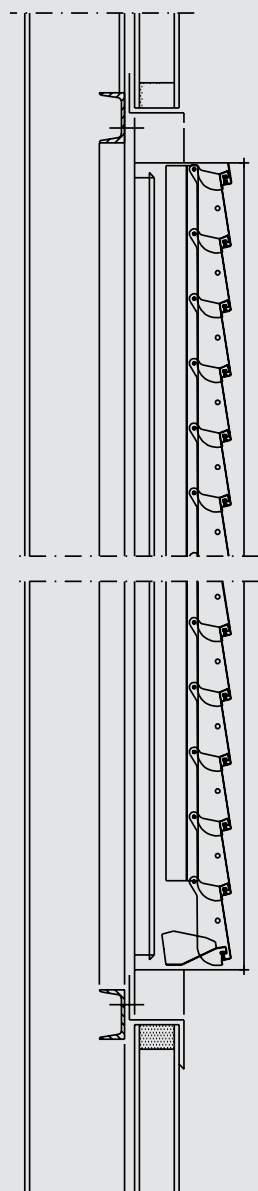
Längsschnitt Lüftungsjalousie Typ FCO
