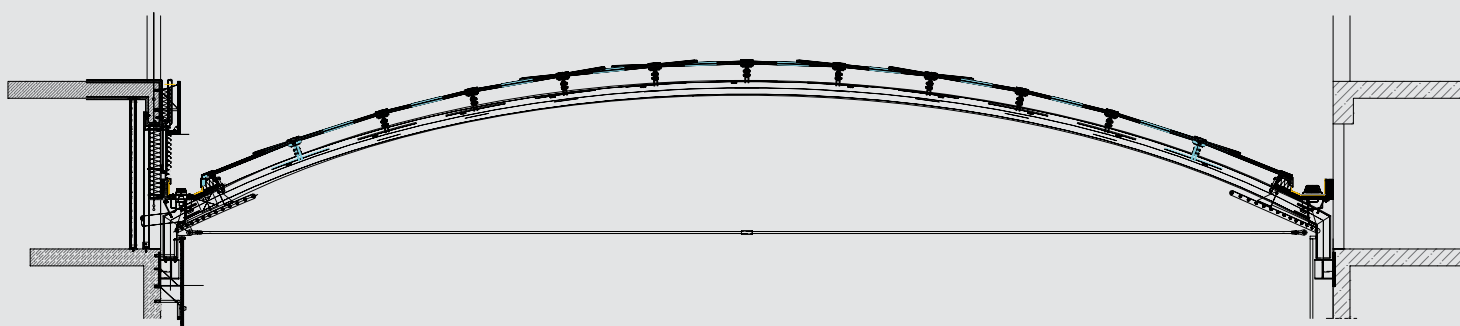
Schnittzeichnung Hallendach
